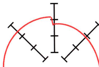
サーボ系の 追従遅れや摩擦
