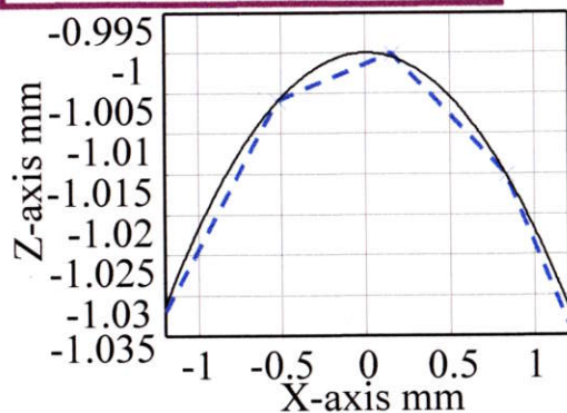
微小線分近似による 誤差(トレランス)
